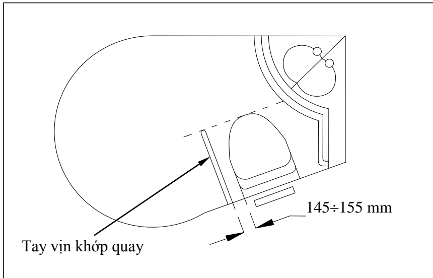
Hình 8 : Sơ đồ bố trí thiết bị vệ sinh tự hoại và tay vịn khớp quay
