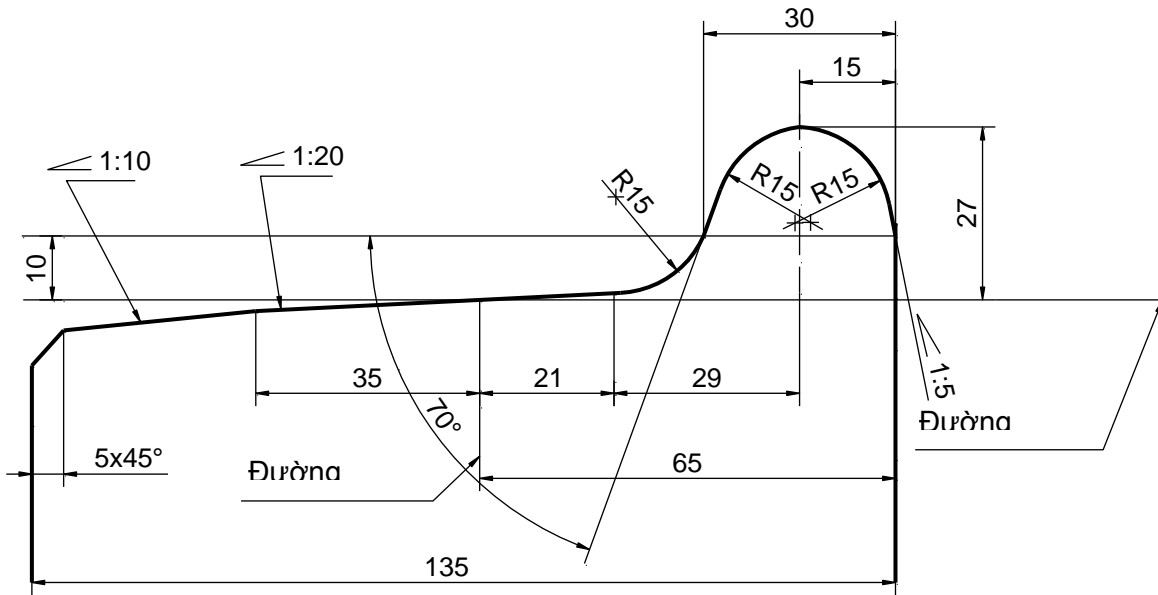
Hình 3. Biên dạng mặt lặn côn khổ đường 1000 mm
